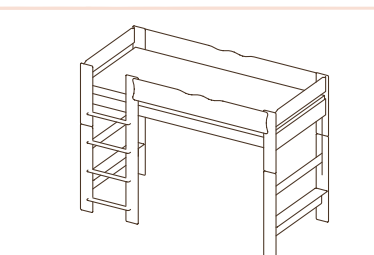
MITTELBETT | letto medio | lit surélevé 147 x 99 x 207 cm (H x B x L) >>MMB09 147 x 109 x 207 cm (H x B x L) >>MMB10
