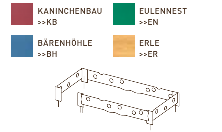
BRÜSTUNGAUFSATZ 2- ODER 4-SEITIG spondina applicata 2 o 4 lati élément de rambarde, 2 ou 4 côtés 26,5 x 99 x 207 cm** (H x B x L) >>BA2 09 26,5 x 109 x 207 cm** (H x B x L) >>BA2 10 26,5 x 99 x 207 cm*** (H x B x L) >>BA4 09 26,5 x 109 x 207 cm*** (H x B x L) >>BA4 10
